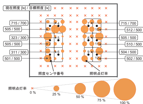
Fig. 3 照度と点灯パターン例 (照明 E, 0.6 m 間隔)
