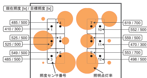
Fig. 2 照度と点灯パターン例 (照明 A, 1.8 m 間隔)
