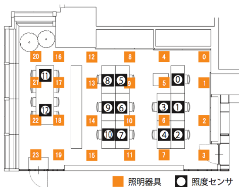
Fig. 1 データ取得環境 (平面図: 7.2 m × 10.1 m)
