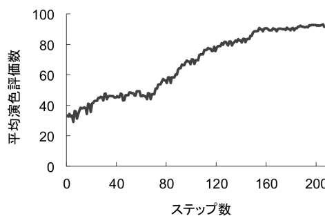
図2: 平均演色評価数変化
