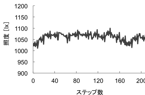
図4: 照度変化
