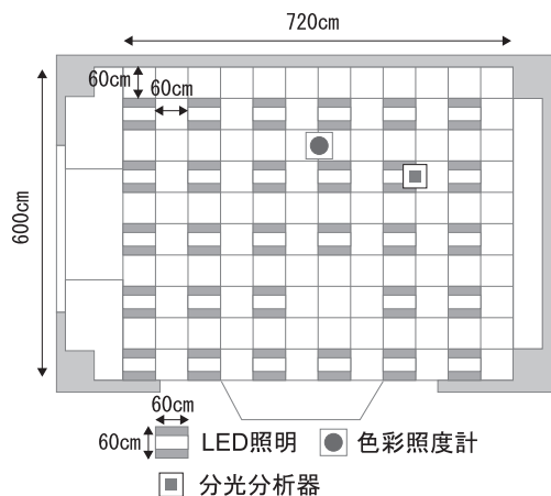
図1: 実験環境 (平面図)
