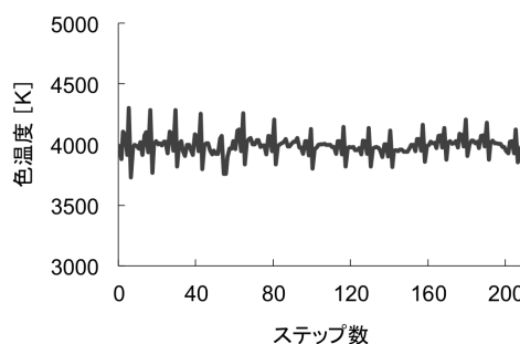
図3: 色温度変化
